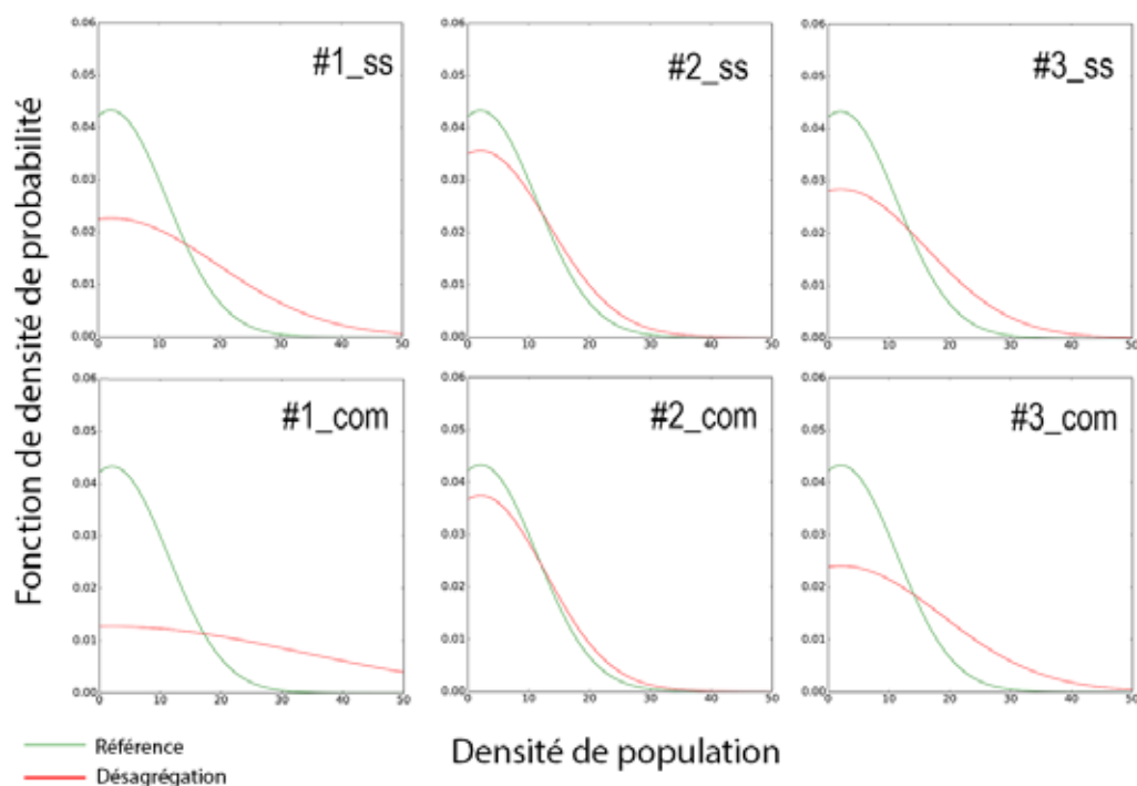
Figure 6 : Fonctions de densité de probabilité du percentile supérieur 99 %
